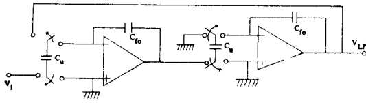
그림 3 프로그램 가능한 2次 SC filter Programmable 2nd order SC filter.
