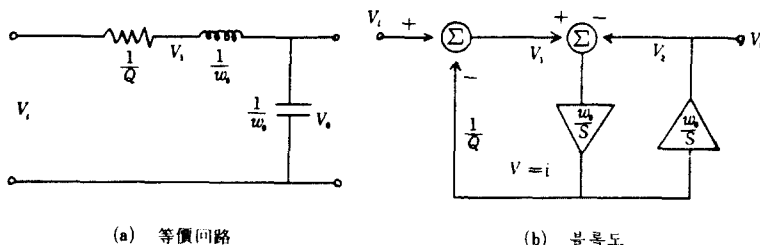
그림 2 Impedance scaling한 回路 Circuit with impedance scaling.
