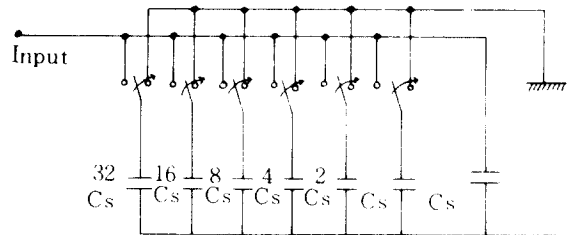
그림 5 6비트 캐패시터 array Six bits capacitor array.
