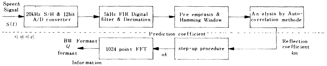
그림 8 Formant 抽出의 블록圖 Block diagram of formant extraction.
