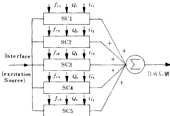
그림 9 並列形의 構成 Parallel structure.
