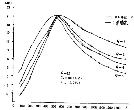
그림12 Q 변화 특성 Characteristics of Q control.
