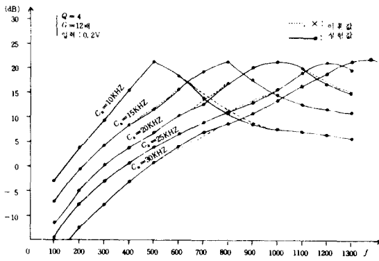
그림11 클럭주파수 변화 특성 Characteristics of clock frequency control.
