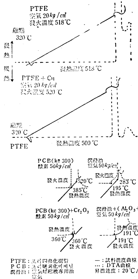
그림 3. 單一有機物에 添加物을 加했을 때의 發火溫度變化
