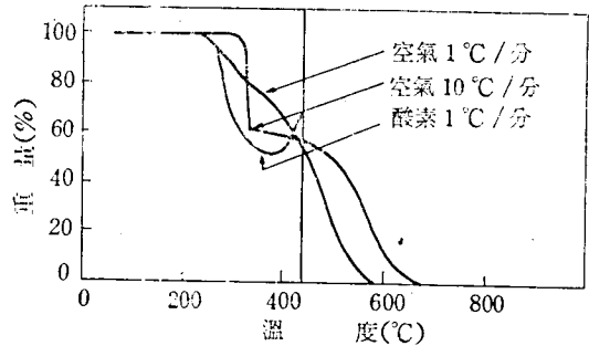
그림 5. 空氣·酸素中의 포리·아크릴로 니트릴의 熱重量
