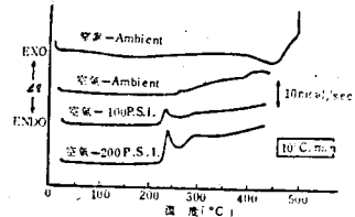
그림 6 示差走査熱分析裝置에 의한 모타油의 測定例
