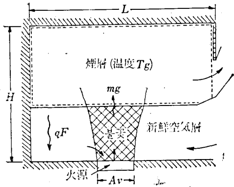
(그림 1) 室火災 Zoning 例
