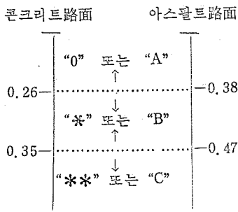
[그림 2] Traction 等級表示
