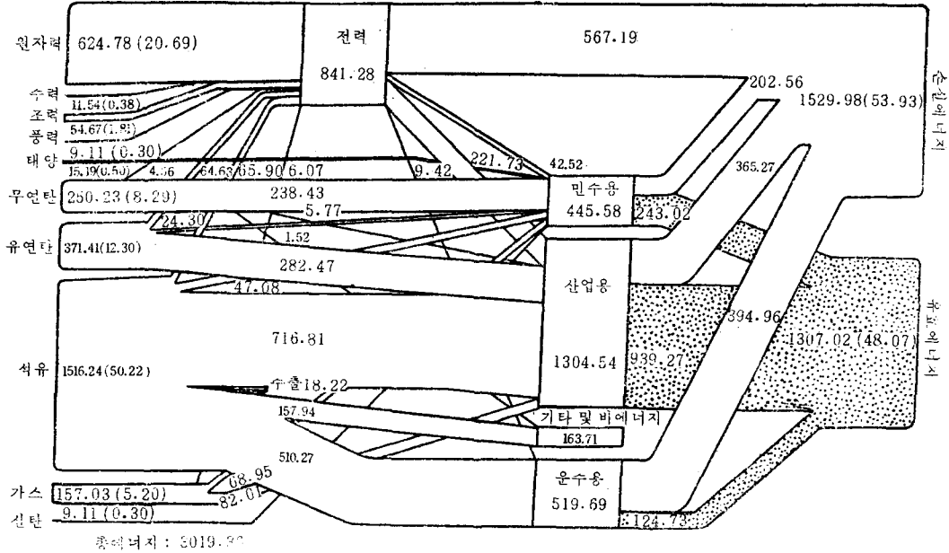
第 7 圖 西紀 2000년의 한국의 에너지 流通構造 展望
