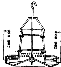
사료통의 단면도
