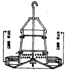
사료통의 단면도
