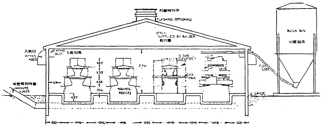
그림 1. 기계화시설의 측면도
