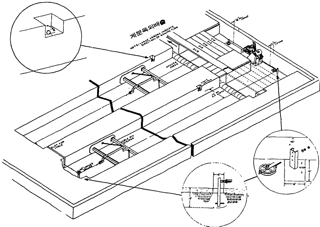
그림 2 : 계분제거 장치(케이블 피트스크래퍼)의 설계
