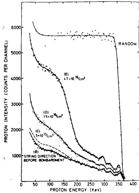
그림 26. <110> 方向에서 各種 線量의 Li 7 이온을 400 keV로 注入한 Si 에 random 및 <110> 方向에서 背面散亂시킨 H + 의 spectra (Gibson)
