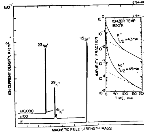
그림 2. 表面이온化型 ion source에서 생긴 ion beam의 質量 spectrum. (Wilson)
