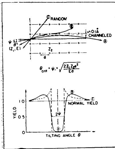
그림 18. 上圖는 加速된 荷電粒子의 運動이 結晶格子에 미치는 影響, Channeling 효과 下圖는 散亂 효과의 角度依存性을 表示했다(Eriksson).
