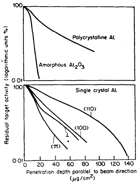
그림 14. 無定形 Al 2 O 3 와 Channeling 現象을 나타낸 多 및 單結晶 Al에 40 keV의 Kr 85 를 衝擊시켰을 때의 積分型射程曲線. (Piercy 等)
