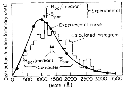
그림 11. Bohr potential 을 사용한 分布曲線의 理論과 Davies 等이 實驗한 結果를 比較한 그림
