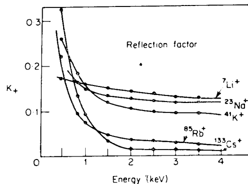
그림 6. a. Mo 表面에 Li + , Na + , K + , Rb + 및 Cs + 이온의 에너지를 變해가면서 衝擊시켰을 때의 각종 이온 反射率 (Brunnee)
