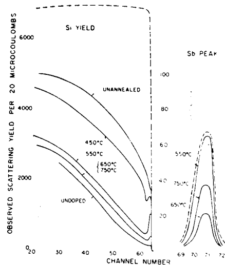
그림 24. 各種 燒鈍溫度에 따른 試料 Si 面의 H + 에 의한 背面散亂 spectra. (Eriksson 等)
