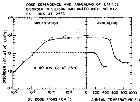
그림 28. 結晶의 disorder(그림 26과 같은 形의 그림에서 測定함)와 40 keV의 Sb 및 Ga 이온으로 Si 結晶을 衝擊하였을 때 그 燒純溫度의 測定 (Eriksson 等)
