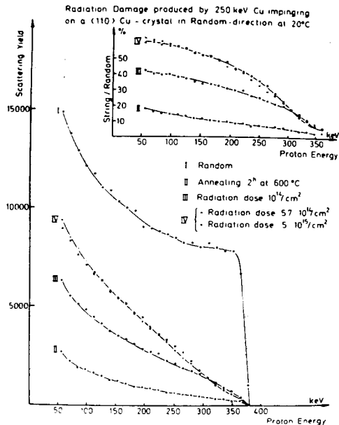
그림 23. Random 方向에서 注入量에 따른 損傷의 程度를 보여준 H + 의 背面散亂스펙트럼. (Andersen)
