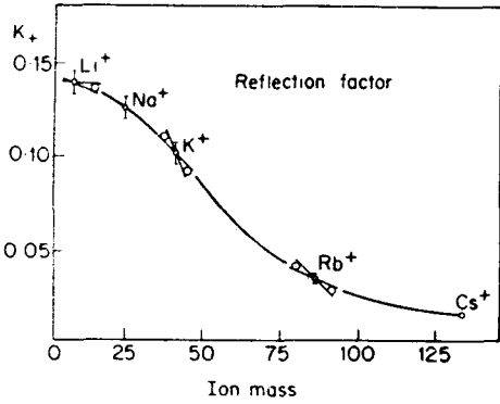
그림 6. b. Mo 表面에 대한 이온 質量에 따른 反射率의 變化(Brunnee)
