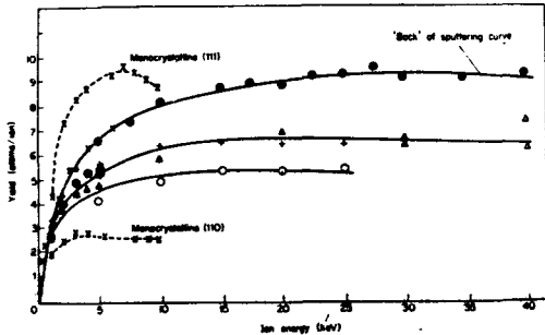
그림 7. a. Ar + 이온의 에너지를 變해가면서 Cu 標 衝擊時 스파터링 收率의 變化(Rol 等)
