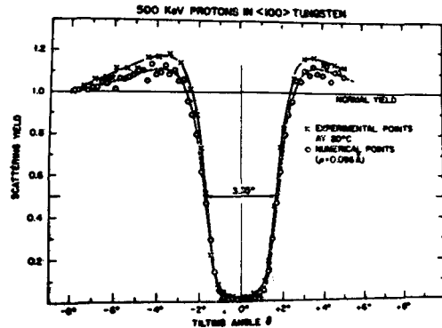
그림 19. W <100> 에서의 背面散亂 陽性子의 角度依存性을 보인 그림이며 이때 入射에너지는 0.5 MeV (20°C). x實驗, (Andersen) o理論(Lindhard).
