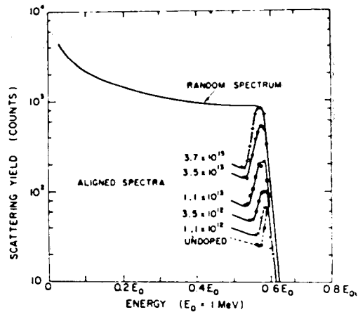
그림 27. Si 單結晶面에서 背面散亂된 1 MeV 의 He 이온의 spectra (Davies 等)
