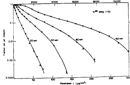
그림 15. Kr 85 의 에너지를 20~160 keV로 變하면서 Al <110> 方位로 衝擊시켰을 때의 滲透(Piercy 等)
