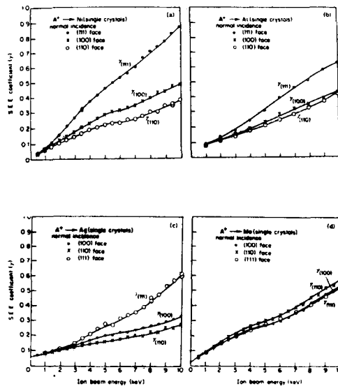
그림 8. 0~10 keV의 Ar + 이온을 Ni, Al, Ag 및 Mo 標의에 衝擊시켰을 때의 2次電子收率 γ의 變化(Carlston 等)
