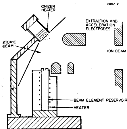
그림 1. 表面이온化型 ion source (Wilson)
