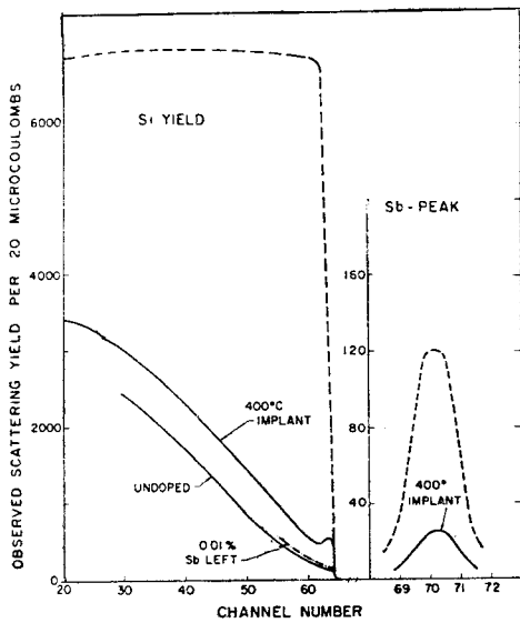
그림 25. 400°C의 “hot implant”를 實施했을 경우에는 別途 post annealing 이 必要없을 程度로 損傷이 回復된다는 事實을 보여준 H + 의 背面散亂 spectra. (Eriksson)
