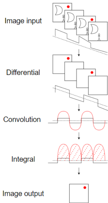
그림 1. 필터의 구조도
