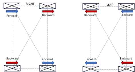
(그림 1) 평행 주行的 조향과 구동 방향
