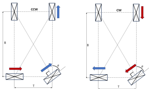
(그림 3) 축회전 회전의 조향과 구동 방향
