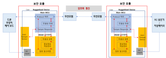
(그림 3) 드론과 지상간 보안모듈의 적용 예.
