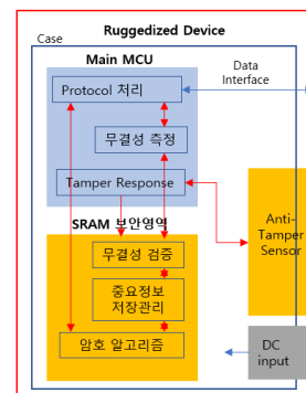
(그림 1) 보안모듈의 SRAM 보안영역 구성도.
