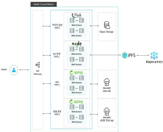
[그림 1] 애플리케이션 구성도
