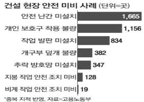
그림 1. 건설현장 안전 미비 사례
