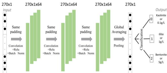
(그림 2) 본 실험에서 사용된 합성곱 신경망 모식도
