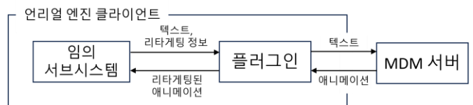
<그림 1> 애니메이션 생성 플러그인 동작 개요
