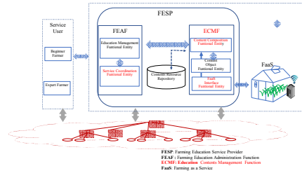
그림 2. 스마트 농업 교육서비스 참조 구조
