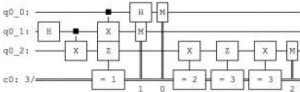
(그림 1) Qiskit 켄텀 텔레포테이션 회로
