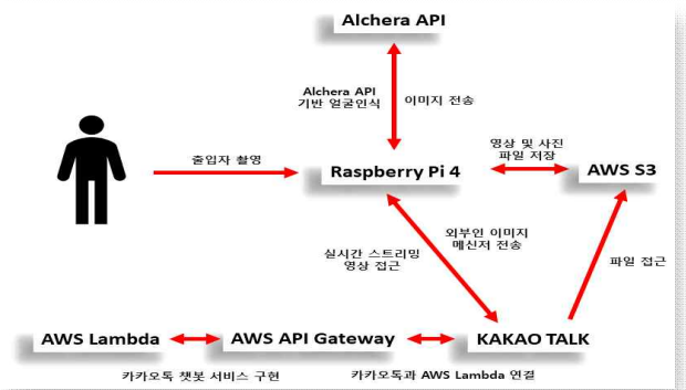
<그림 1> 비대면 출입자 모니터링 전체 블록도
