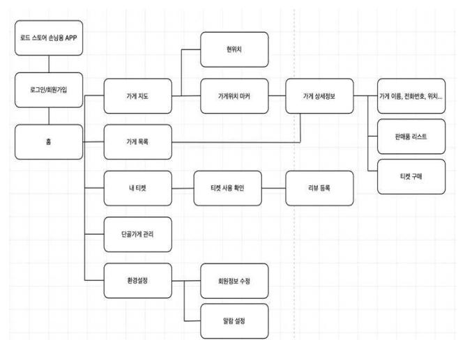
(그림 3) 일반 손님용 어플리케이션 구조도
