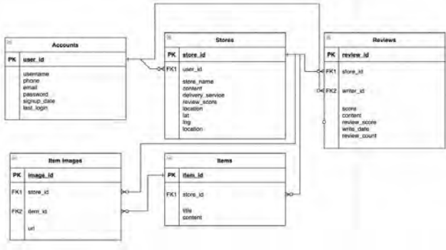
(그림 4) 데이터베이스 관계도
