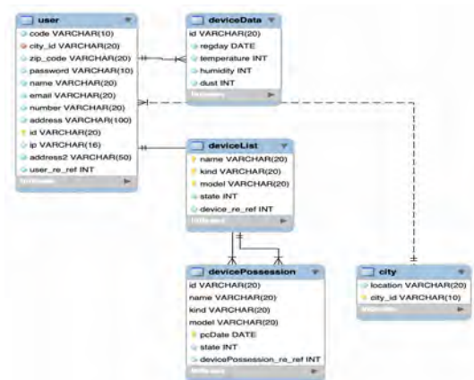
그림(5) 웹 사이트 ER 다이어그램
