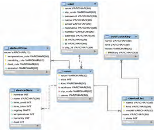
그림(7) 스마트홈의 ER 다이어그램
