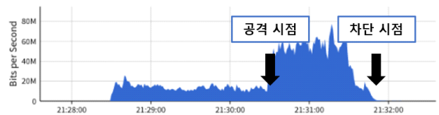
(그림 5) Port 기반 차단 기법 적용 결과
