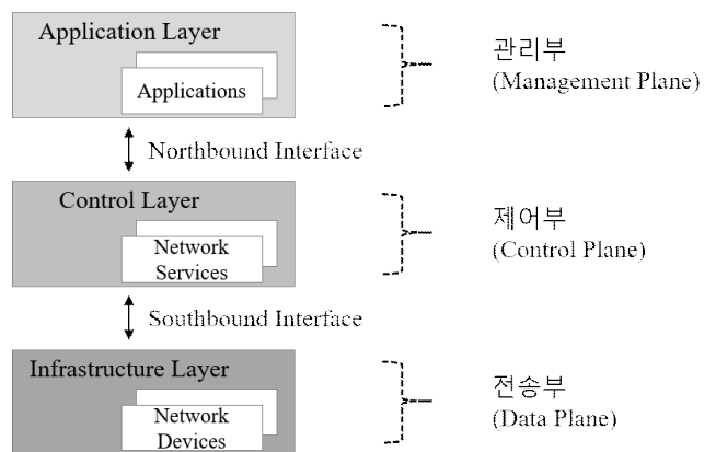
(그림 1) SDN의 구조
