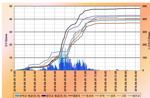
(2) 10분 누가강우량곡선(2018.08.28~08.30)
