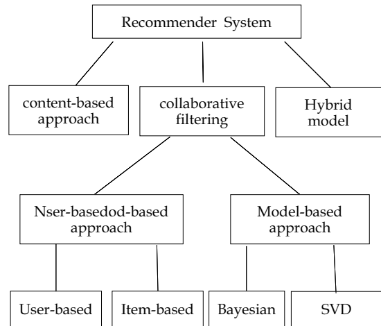
그림 1. 추천시스템 분류
