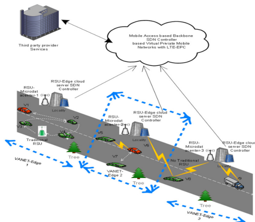
그림 1. Overview of SDCVN framework.
