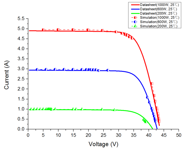
그림 7. Hybrid Control을 이용한 SAS Simulation (PV panel : SQ160PC)
