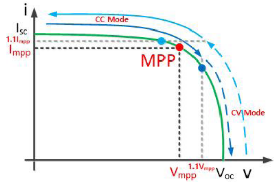
그림 5. Hybrid Controller
