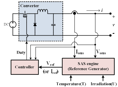
그림 1. Solar Array Simulator
