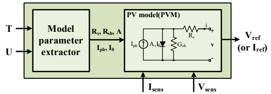
그림 2. PV model-based SAS Engine
