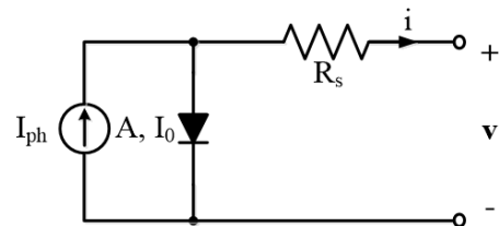
그림 3. Simplified Single Diode 모델
