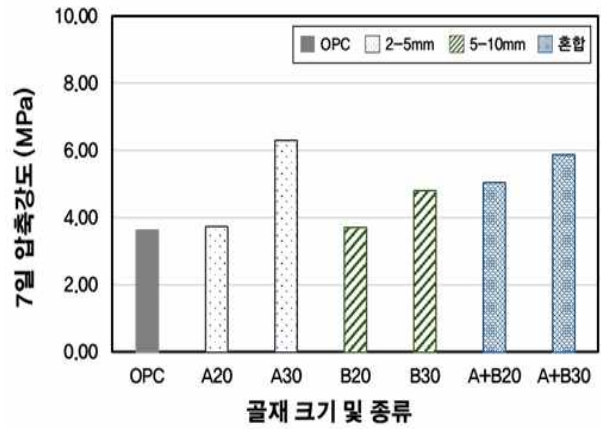
그림 2. 7일 압축강도
