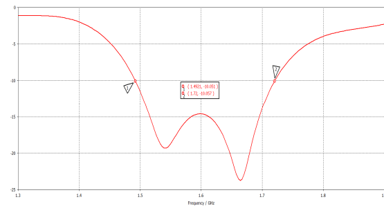
그림 2. 반사계수
