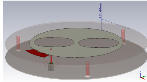
그림 1. 제안된 안테나 구조
