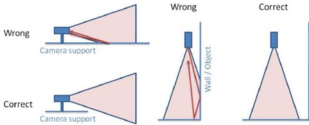
그림 6. ToF 카메라 배치 방법
