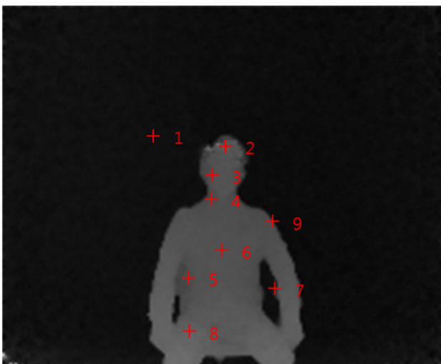
그림 12. 사람 깊이맵
