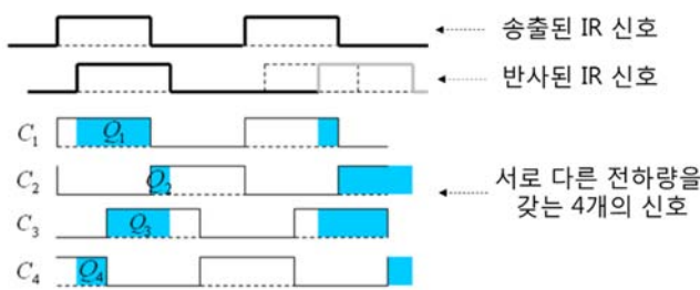
그림 2. 위상차를 이용한 깊이맵 계산
