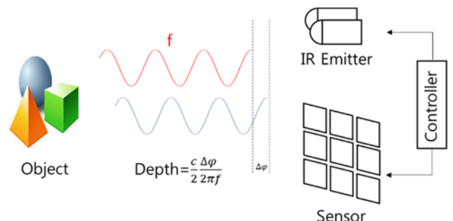
그림 1. 깊이 카메라 원리
