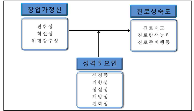
<그림2> 연구모형
