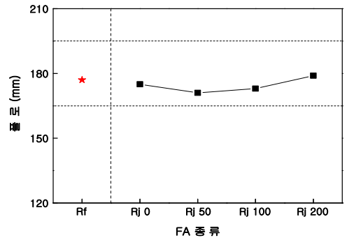
그림 1. FA 종류 변화에 따른 플로
