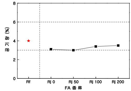
그림 2. FA 종류 변화에 따른 공기량
