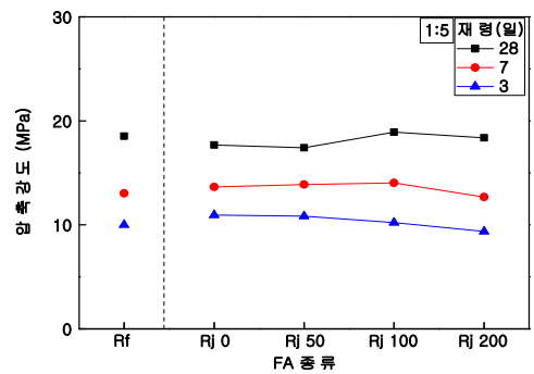
그림 3. FA 종류 변화에 따른 압축강도
