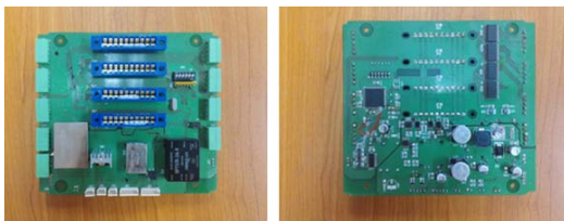
그림 3. 개발된 통신 게이트웨이 메인 보드 Fig. 3. The Development of Communication Gateway Main Board
