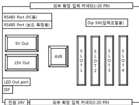
그림 2. 통신 게이트웨이 메인 보드 디자인 Fig. 2. The Design of Communication Gateway Main Board
