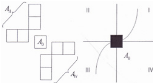
a) 격자형 직각 좌표계 b) I-III형 에지의 예 그림 1. 에지 검출 알고리즘에 사용된 창의 구성
