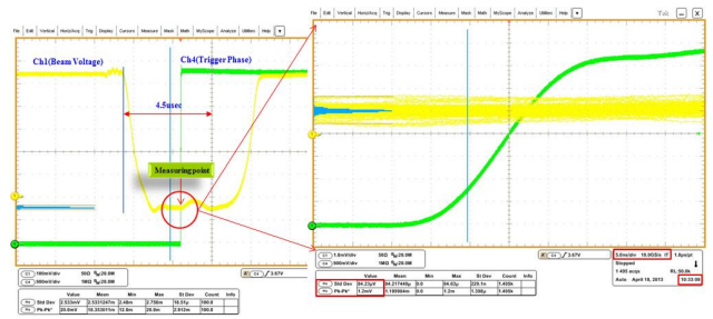
<그림 6> 빔전압 Stability 측정 파형
