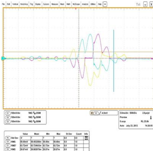
<그림 9> 인버터형 고정밀 고전압 전원장치 전류 파형
