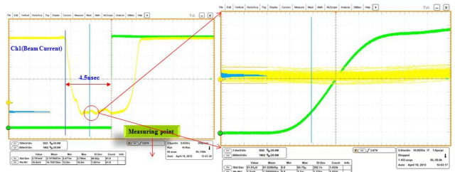
<그림 7> 빔전류 Stability 측정 파형
