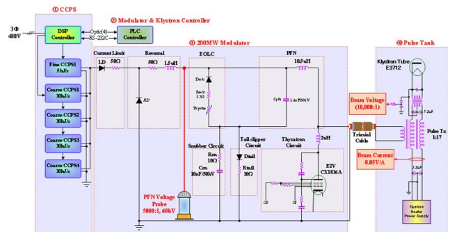
〈그림 1〉 고정밀 인버터 전원공급장치를 사용한 펄스 모듈레이터 회로
