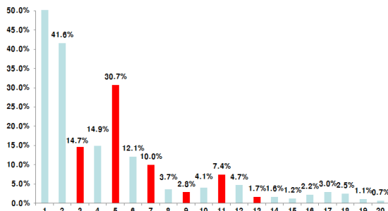
<그림 10> 입력 전원측 고조파 전류 스펙트럼[%]
