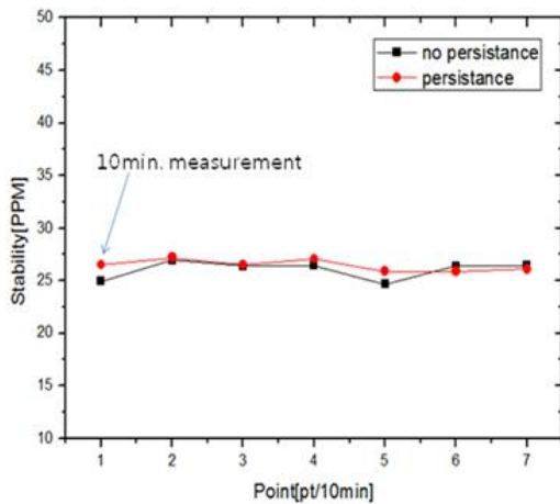
<그림 8> 빔전압 Stability 연속 측정 데이터
