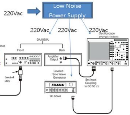
<그림 5> Stability 측정용 setup
