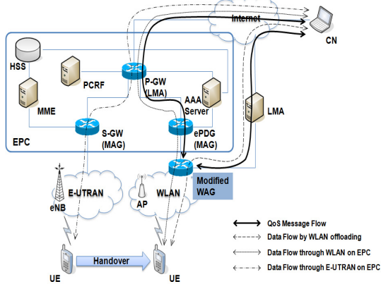
그림 1. 제안한 트래픽 경로 선택 기법
