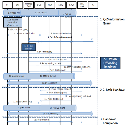
그림 2. 제안한 기법의 핸드오버 절차
