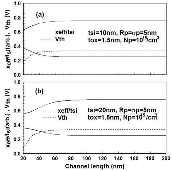
그림 2. 채널길이의 변화에 따른 문턱전압 및 전도중심의 변화 (a) 채널두께가 10nm일 때 (b) 채널두께가 20nm일 때
