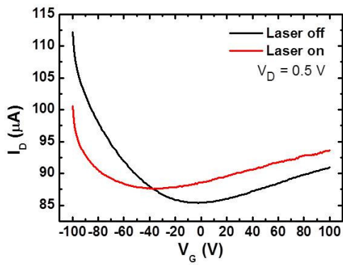
그림1. 그래핀 광소자의 I_D - V_G 광응답 곡선. 레이저가 채널에 조사되었을 경우 그래프가 왼쪽으로 이동한다.
