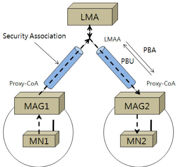
(그림 1) PMIPv6 동작 과정
