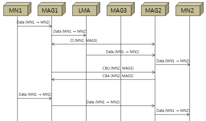
(그림 4) MAG간의 이동성을 보장하는 경로 최적화 설정 과정
