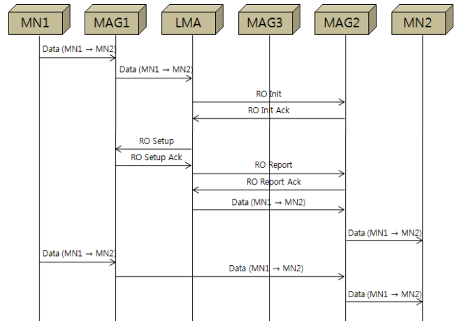
(그림 2) Liebsch Proxy Mode에서의 경로 최적화 설정 과정
