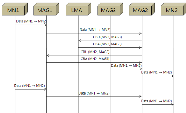
(그림 3) Dutta의 경로 최적화 설정 과정
