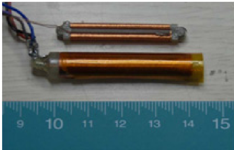
그림 1. 제작된 flux-gate센서의 사진.
