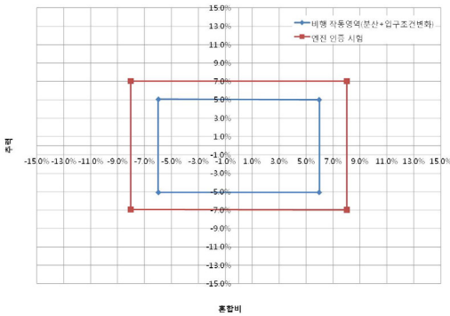
Fig.1 엔진 비행작동영역과 엔진 인증 시험 영역
