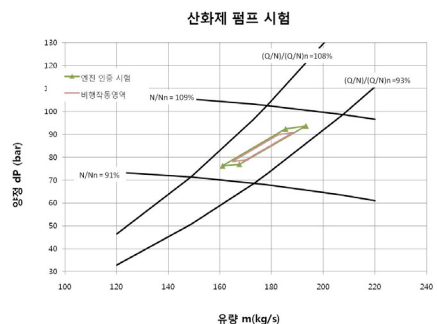
Fig. 8 산화제 펌프 시험영역 요구조건
