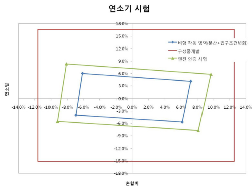
Fig. 3 연소기 시험 영역 요구조건 (설계점 대비)
