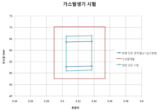
Fig. 6 가스발생기 시험 영역 요구조건
