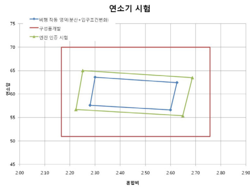
Fig. 4 연소기 시험 영역 요구조건
