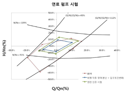
Fig. 9 연료펌프 시험 영역과 해외사례비교
