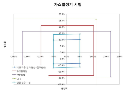
Fig. 5 가스발생기 시험 영역 요구조건과 해외 사례
