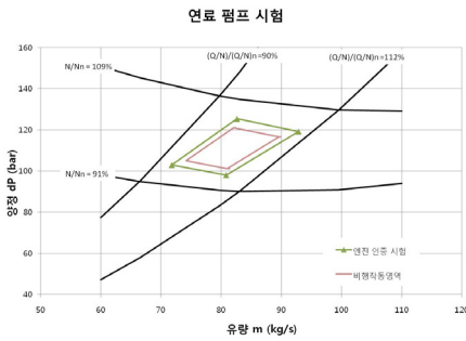
Fig. 10 연료펌프 시험 영역 요구조건
