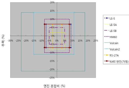
Fig. 2 엔진 시험 영역 해외 사례 비교
