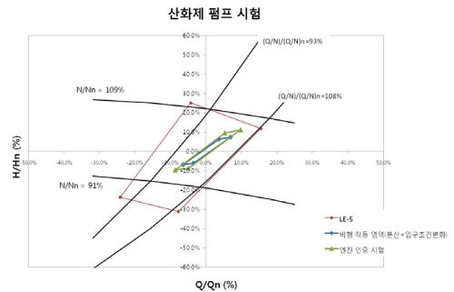
Fig. 7 산화제 펌프 시험 영역과 해외사례비교
