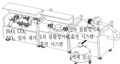
그림. 2. Equipment Assembly
