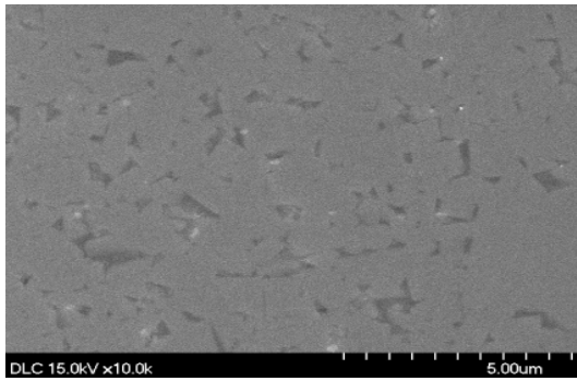
(b) DLC 코팅 후 WC 코어 표면 SEM 사진
