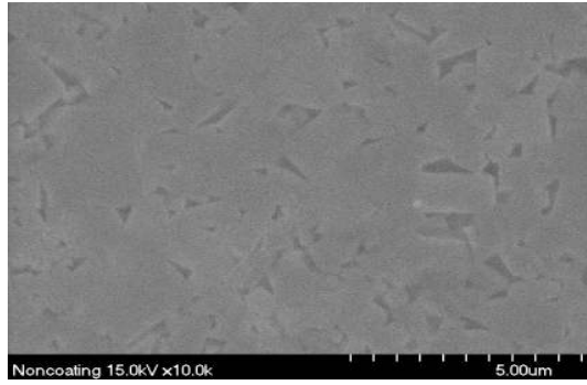
(a) DLC 코팅 전 WC 코어 표면 SEM 사진
