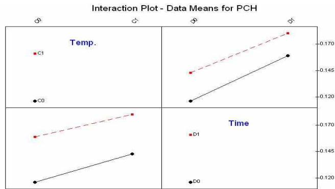
[그림 6] 탈기 공정에서 PCH에 대한 교호작용
