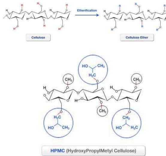
[그림 1] HPMC 합성 메카니즘
