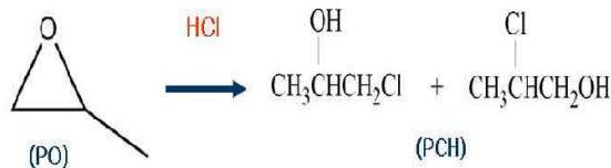
[그림 4] PCH 생성 메카니즘
