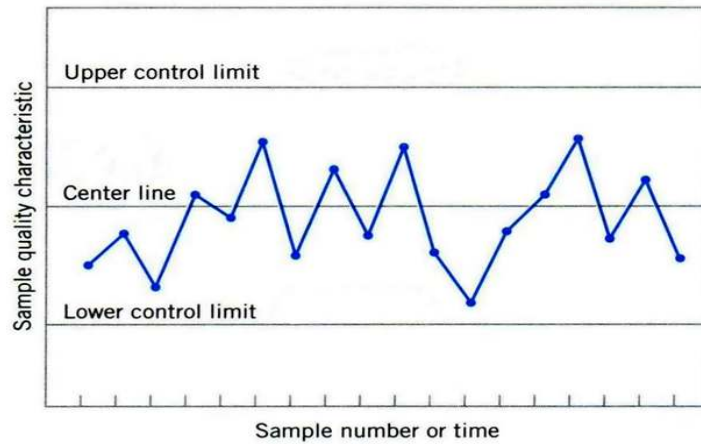
[그림 1-1] 일반적인 슈와트(Shewhart)관리도
