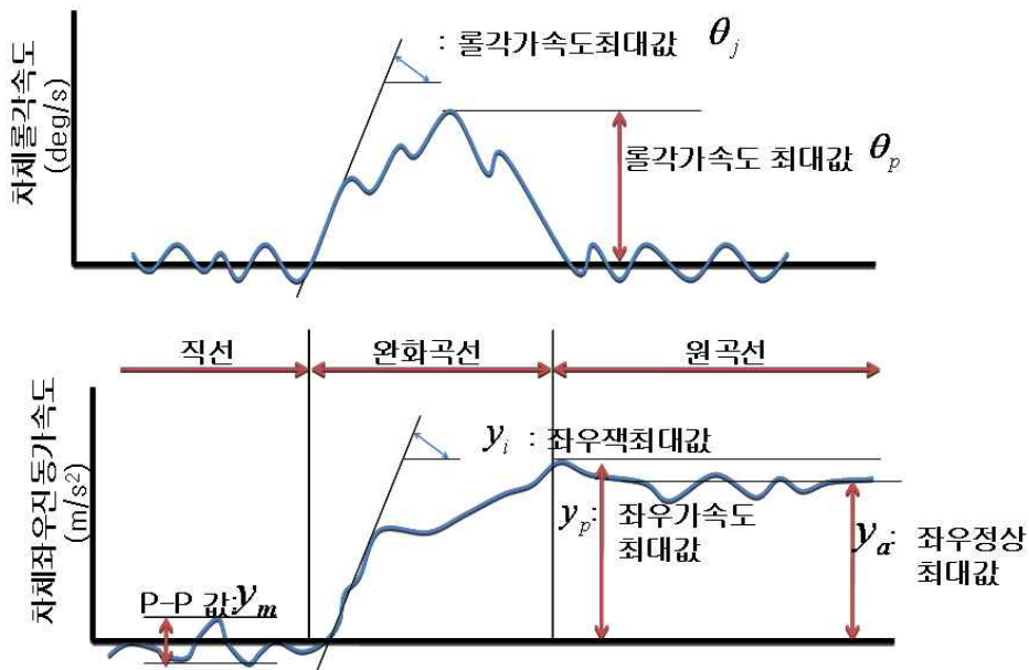
그림 2 틸팅 차량의 곡선 주행시의 승차감을 나타내기 위한 주요 지표
