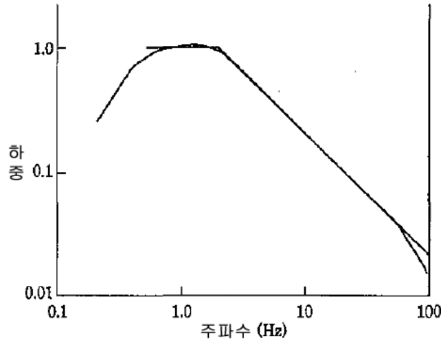
그림 3 주파수 보정 필터(Wd) 6)
