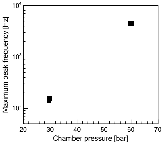
Fig. 7 최대 파워스펙트럼에서의 주파수
