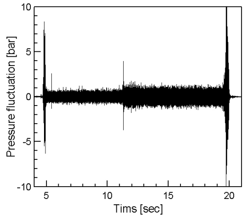
Fig. 4 첫 번째 연소시험의 필터링 된 압력 섭동
