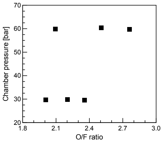
Fig. 3 혼합비 대 연소실 압력
