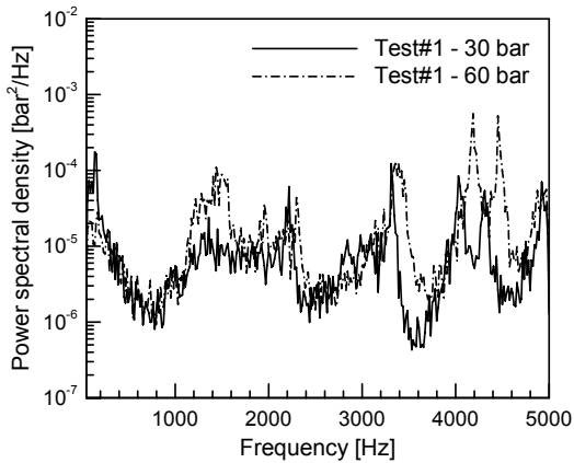
Fig. 6 압력 섭동의 파워스펙트럼
