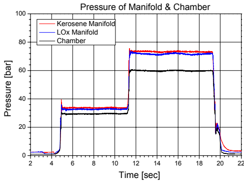
Fig. 2 매니폴드 및 연소실 압력
