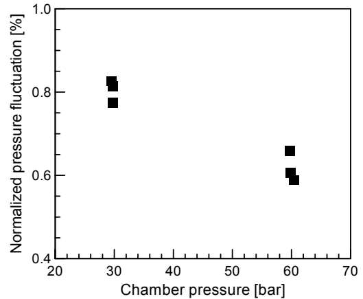
Fig. 8 정규화된 압력 섭동 RMS 값
