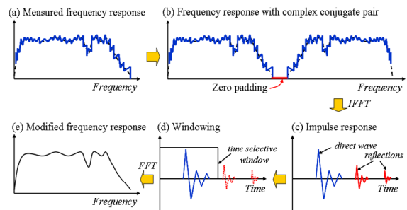
Fig 2. 신호의 선택적 분리와 처리과정
