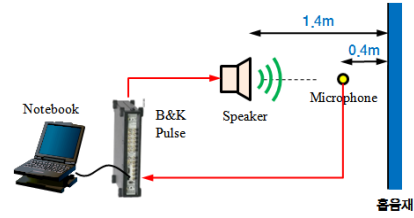
Fig 5. In-situ 시스템 개략도
