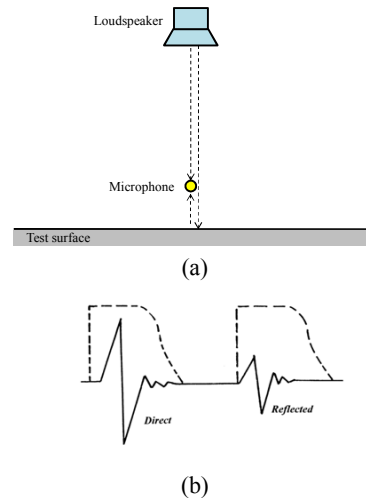
Fig 1. (a) 반사법의 원리, (b) 임펄스응답 구성
