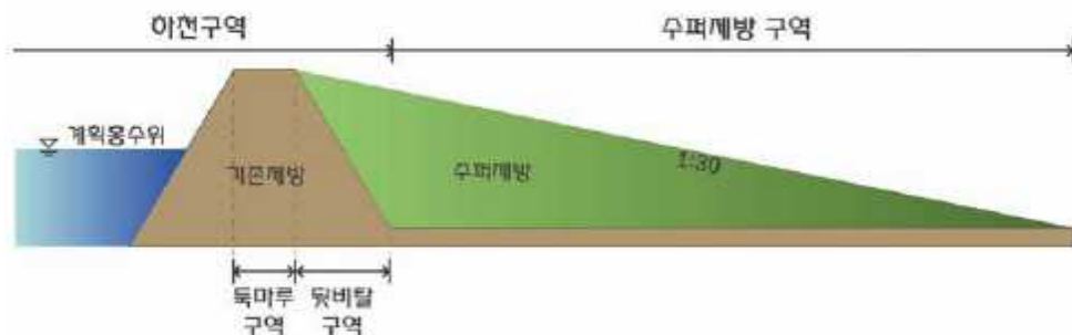
그림 3. 수퍼제방의 구역 구분
