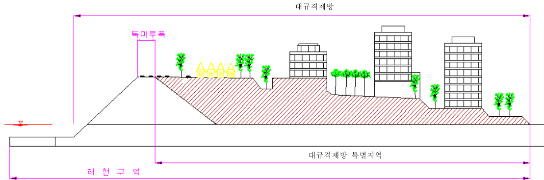
그림 2. 대규모제방의 형태(하천설계기준·해설, 2009)
