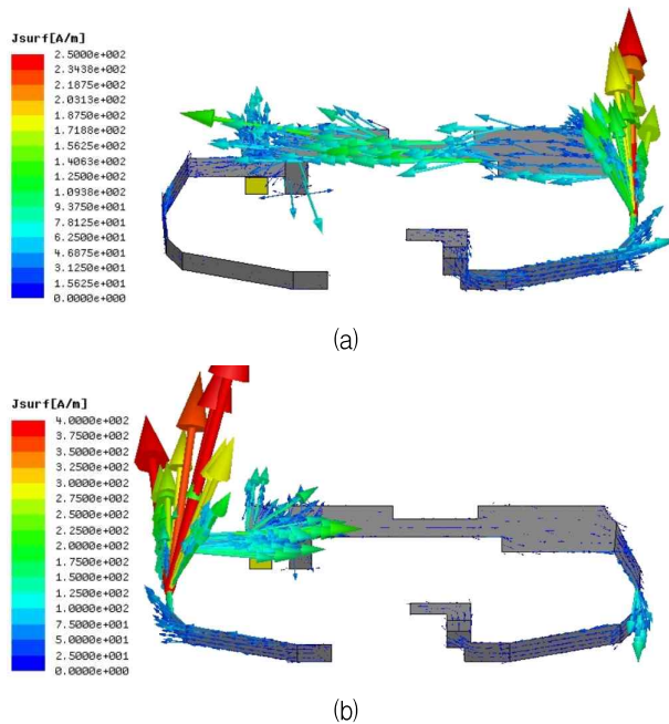
<그림 3> 대역별 전류밀도 시뮬레이션 이론데이터 (a) GSM, (b) DCS/USPCS/WCDMA
