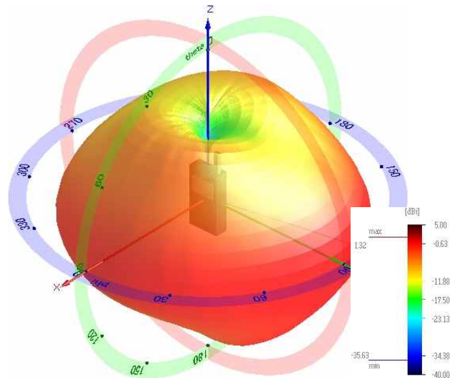
<그림 9> 제작한 안테나의 GSM대역 3D방사패턴
