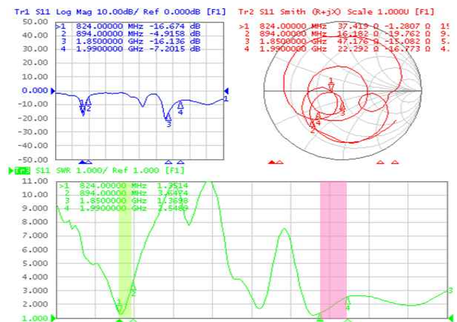
<그림 6> 기존안테나의 반사손실, VSWR, 스미스차트
