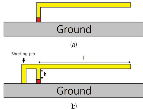
<그림 1> 안테나의 구조 (a) ILA (b) IFA
