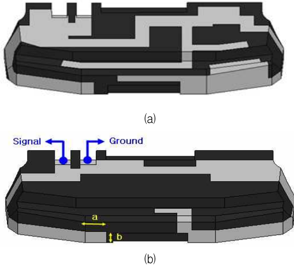
<그림 2> 시뮬레이션 툴로 구현 및 설계 (a) 기존의 안테나, (b) 제안한 안테나
