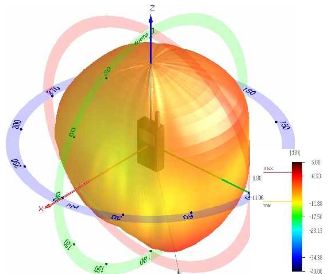
<그림 10> 기존안테나의 DCS/USPCS/WCDMA대역 3D방사패턴
