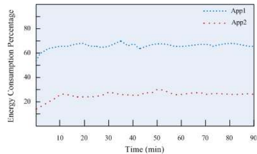
그림 3. 두 응용 프로그램의 에너지 사용량
